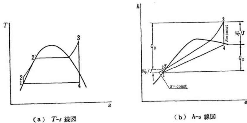
図 5.4 ランキンサイクル
