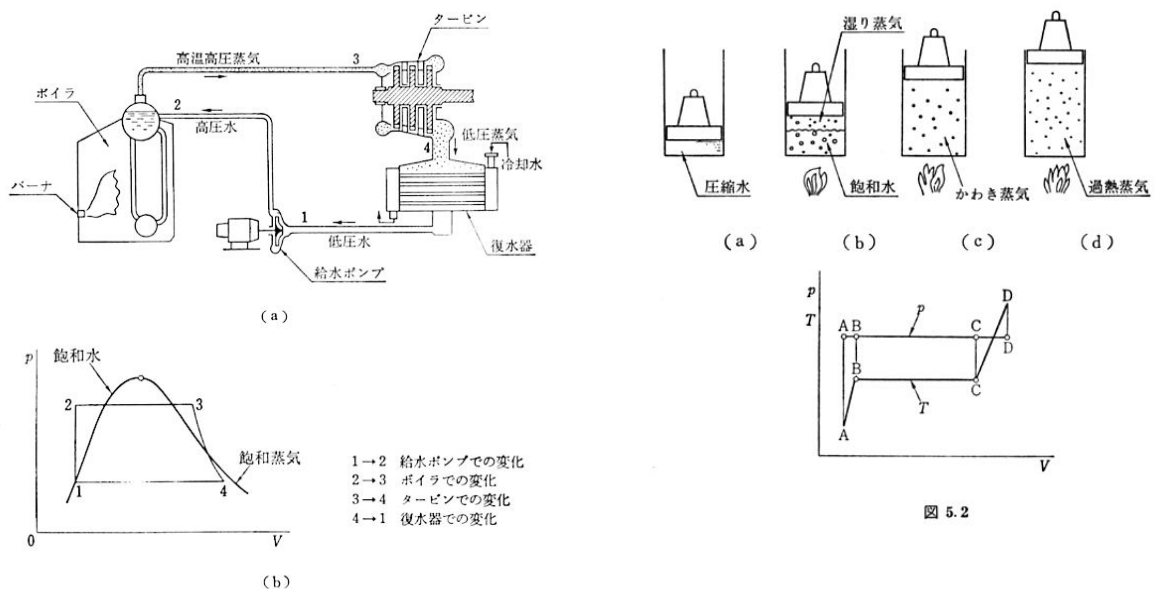
図 5.1 蒸気サイクル
