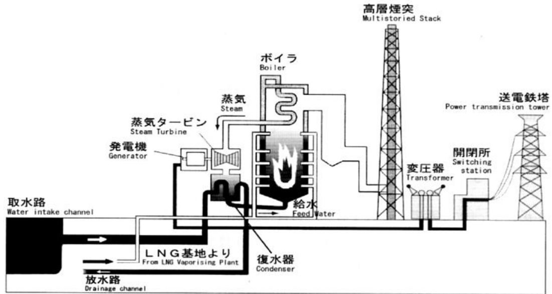
図 9.8 LNG 火力発電所例 (資料提供東北電力株)
