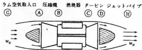
図 4-9 ターボジェットサイクルの配置図
