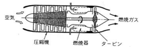
図 4-78 ターボジェットエンジン
