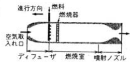
図 4-81 ラムジェットエンジン
