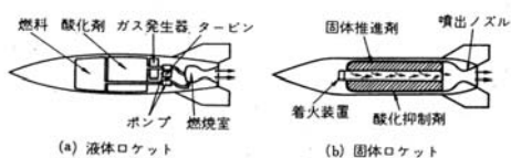
図 4-82 ロケットエンジン
