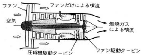
図 4-79 ターボファンエンジン
