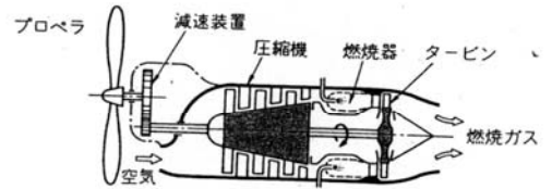
図 4-77 ターボプロップエンジン
