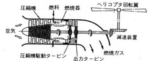
図 4-76 ターボシャフトエンジン
