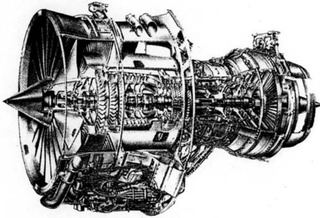
図 4-80 ターボファンエンジン
