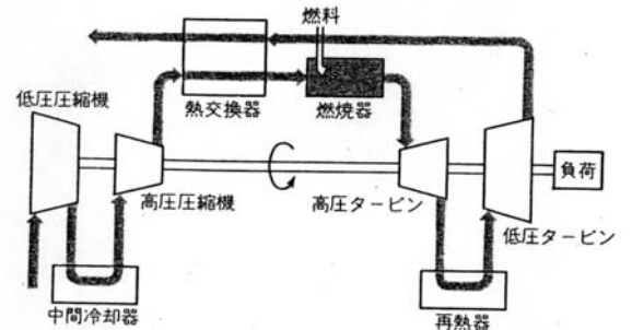
図 4-75 実際のサイクルの例
