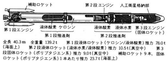
図 4-83 人工衛星打上げ用ロケット (H-I型ロケット (宇宙開発事業団))
