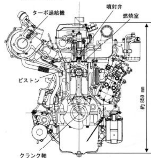
(b) トラック用ディーゼルエンジン (6H-K1, フォワード搭載, いすゞ自動車(株)提供)
