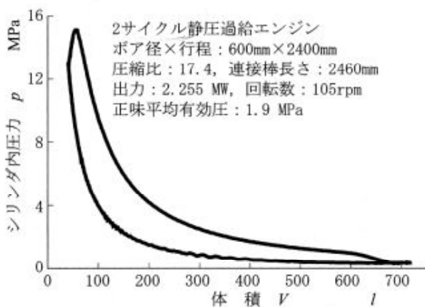
(c) 船用ディーゼルエンジン (S60MC-C, 三井造船(株)提供)
