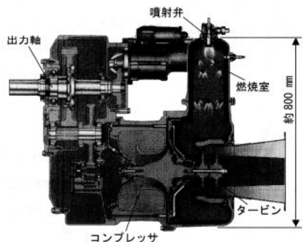
(d) ガスタービンエンジン (ATG-300, 小形発電用, ヤンマーディーゼル(株)提供)
