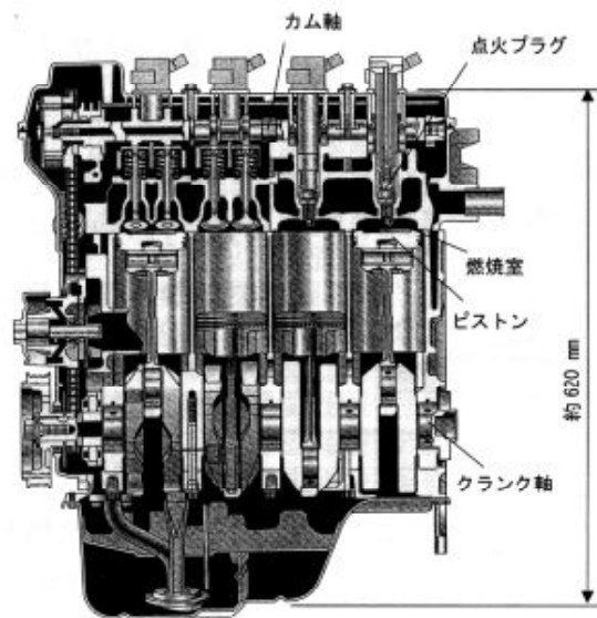
(a) 乗用車用火花点火エンジン (1ZZ-FE, カローラ搭載, トヨタ自動車(株)提供)
