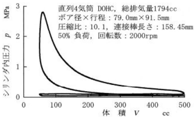
(a) 乗用車用火花点火エンジン (1ZZ-FE, カローラ搭載, トヨタ自動車(株)提供)
